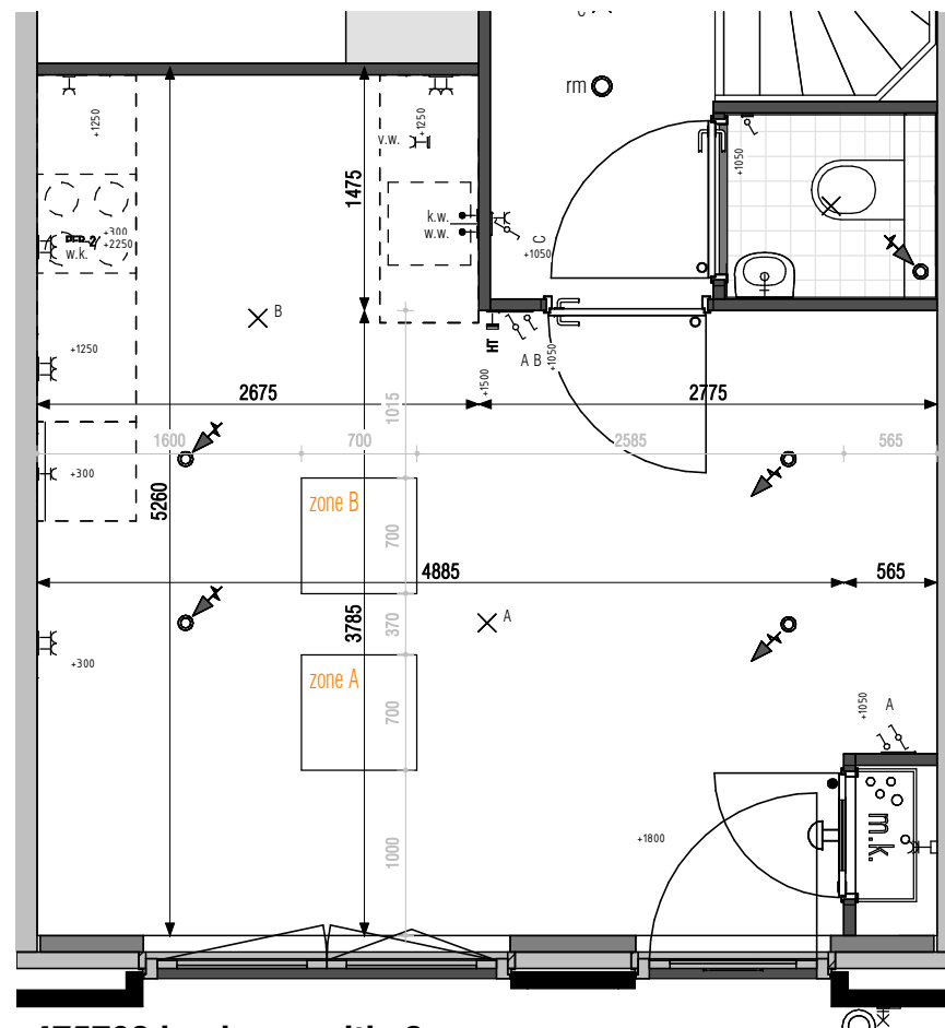
475703 keukenpositie 3 gevel bnrs getekend: 73, 79, 156
