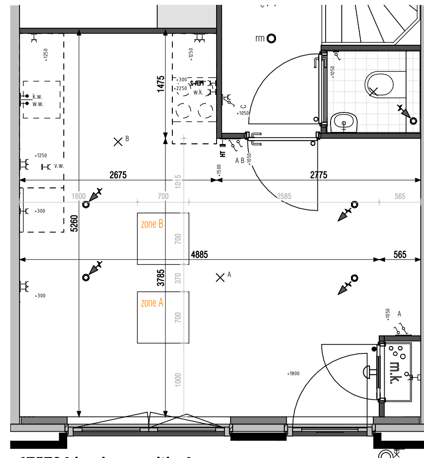
475704 keukenpositie 4 gevel bnrs getekend: 73, 79, 156
