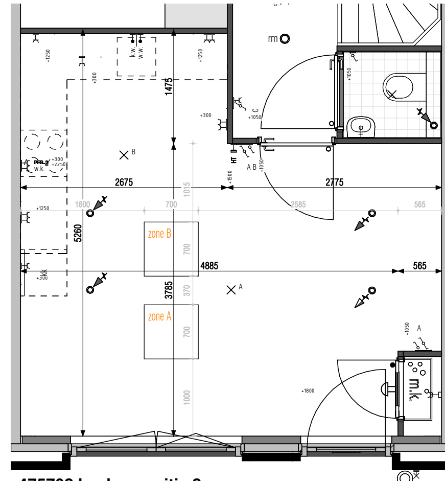
475702 keukenpositie 2 gevel bnrs getekend: 73, 79, 156
