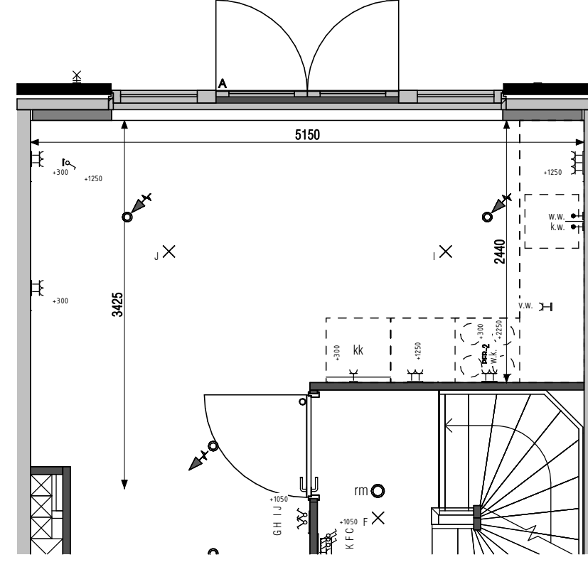
475431 keukenpositie 31 (standaard)
