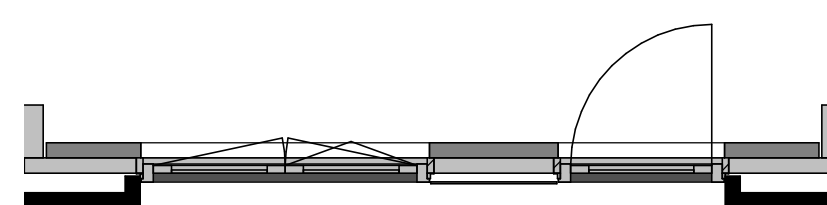
Voorgevel bnrs: 69, 148
