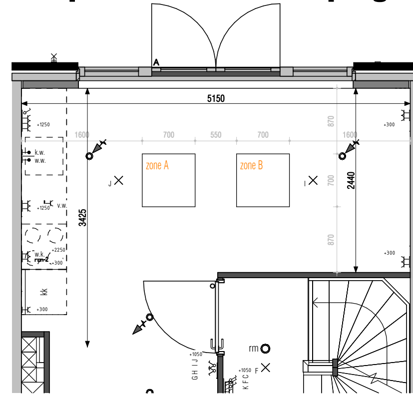
475431 keukenpositie 31 (standaard)
