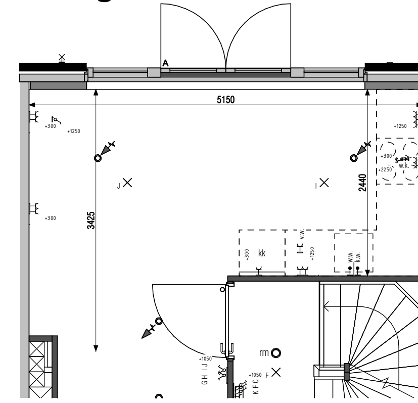
475432 keukenpositie 32
